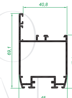
61.2145 Hoja vidrio 45
