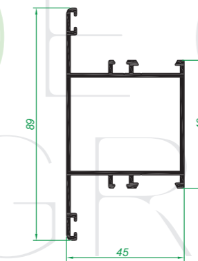
70.3949 Transversal Vidrio
