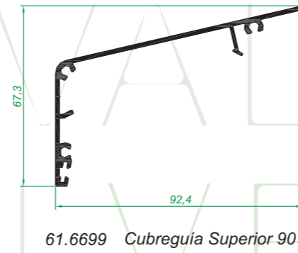
61.6699 Cubreguía Superior 90
