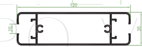
60.758 | Zócalo cerrado 10
