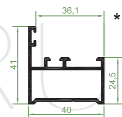
60.651 | Marco Ventana 40
