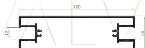
61.808 | Zócalo 120 lamas
