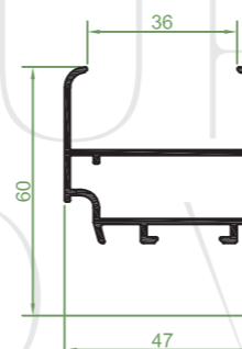
61.802 | Hoja ventana mallorquina
