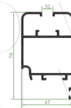
60.772 | Hoja cerrada 10 puerta
