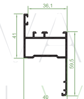
60.671 | Marco 40 con tapajuntas
