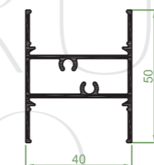
61.810 | Travesaño 50
