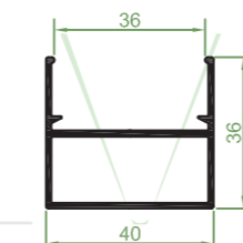
61.809 | Marco fijo 40
