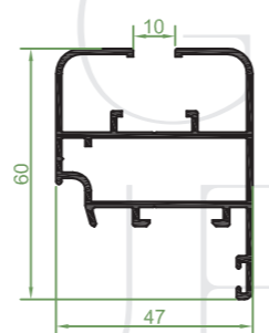
60.652 | Hoja cerrada 10 ventana
