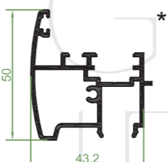
60.655 | Inversor hoja
