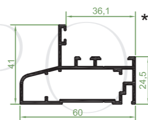
60.661 | Marco Ventana 60
